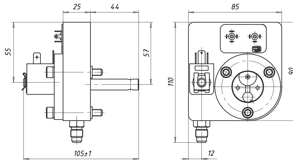
Fig.4. Dimensions
